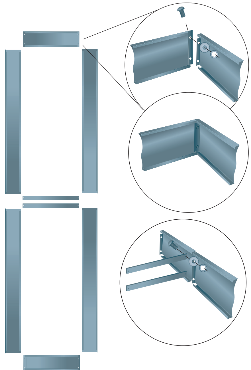
Схема сборки грядки со вставкой
